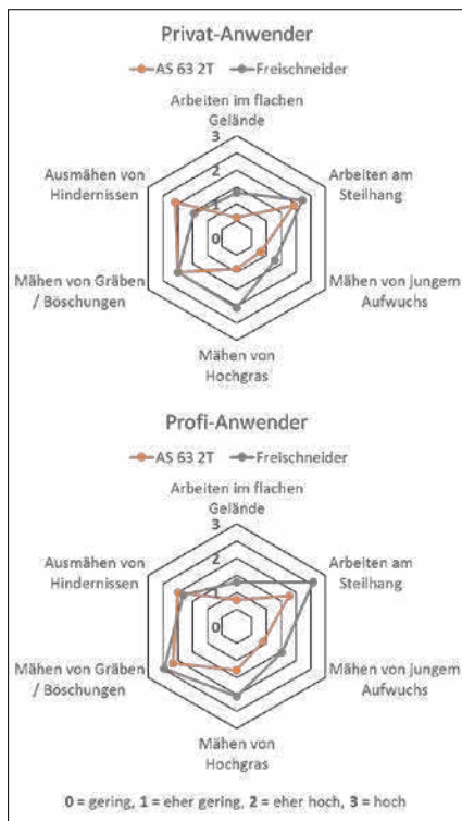
Abb. 8: Bewertung des Kraftaufwands beim Mähen in unterschiedlichem Gelände mit Hochgrasmäher AS 63 2T und Freischneider durch die Anwendergruppen „Privat“ (n=47) und „Prof“ (n=18).
